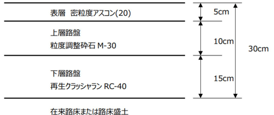
舗装断面構成
