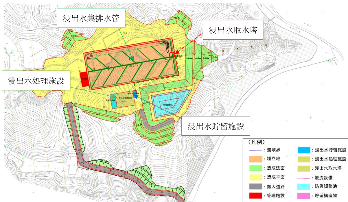
図 10.4.5 浸出水集排水施設配置図
