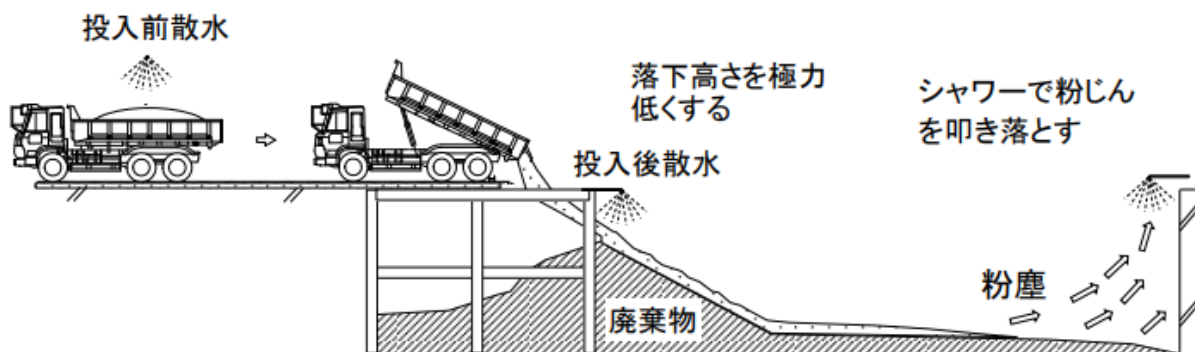
図 7.5.2 ダンピングステージ投入方式
