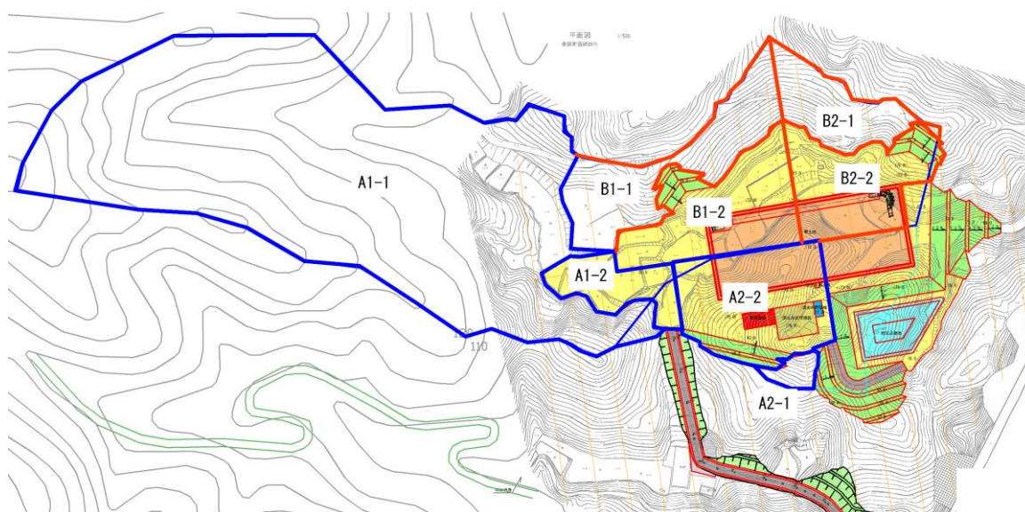
図 10.6.4 集水範囲（左右岸）
