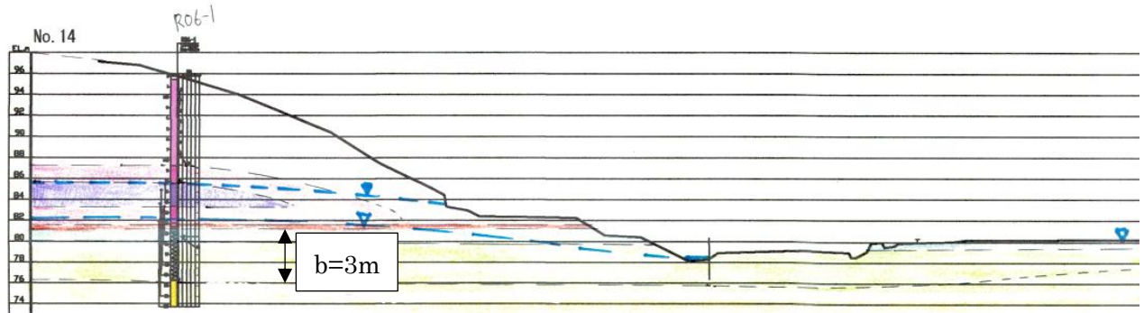
図 10.5.6 No.14 断面図
