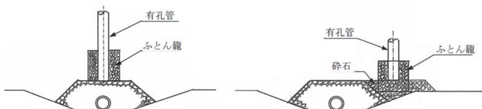
図 10.4.7 豎型集排水管の構造例
