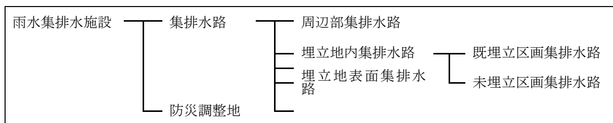
図 10.6.1 雨水集排水施設の分類
