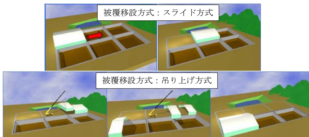
図 7.4.1 区画埋立と被覆施設の移設
