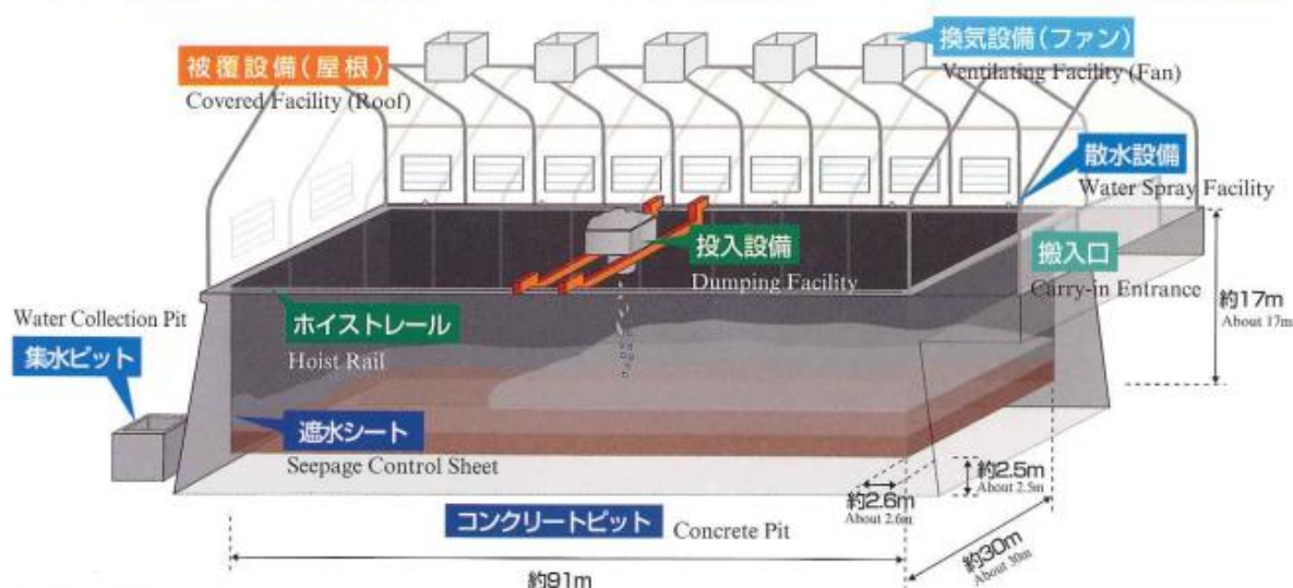
図 7.5.3 機械投入方式
