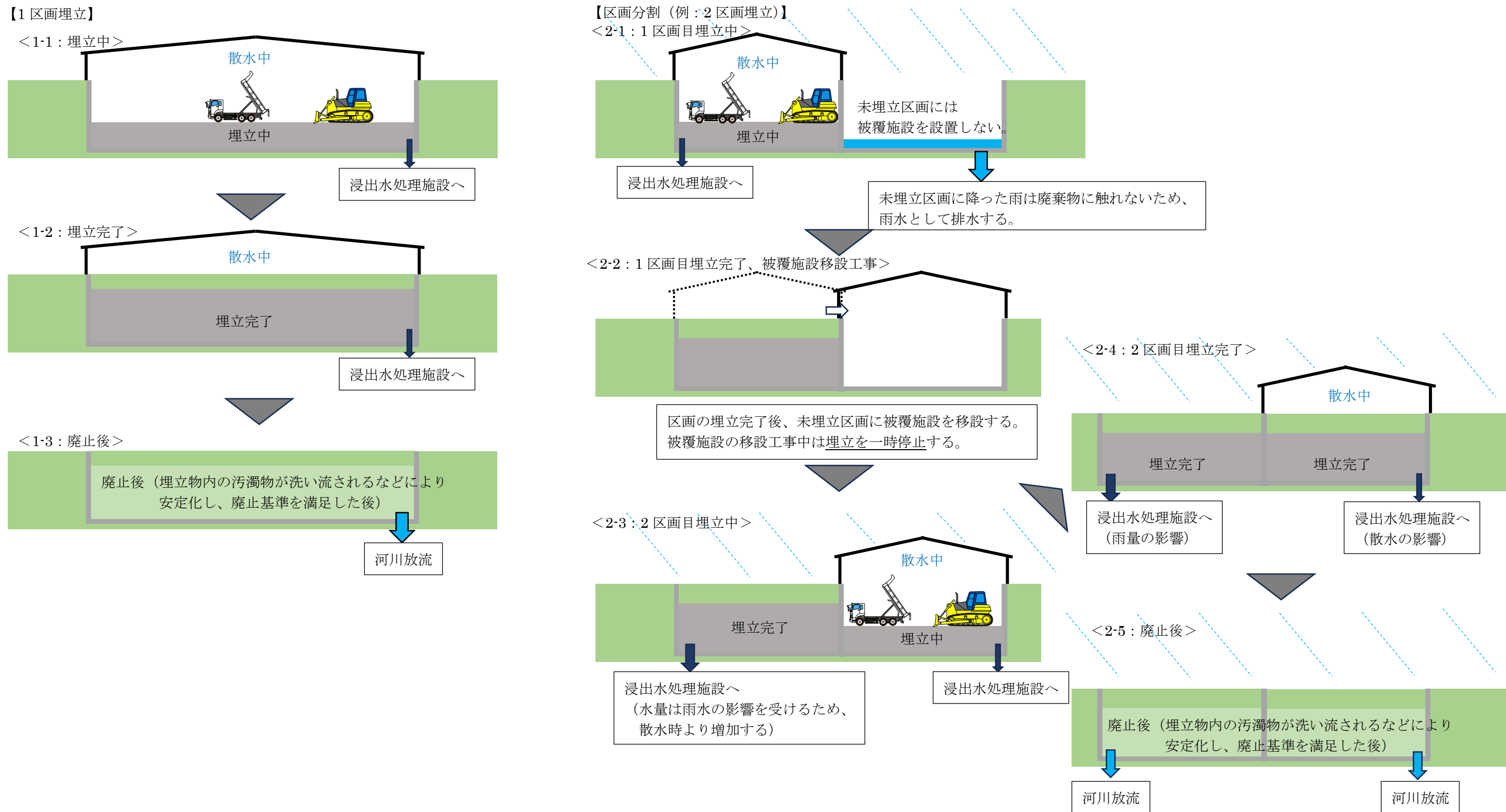
図 7.4.2 区画埋立の有無による埋立順序イメージ図
