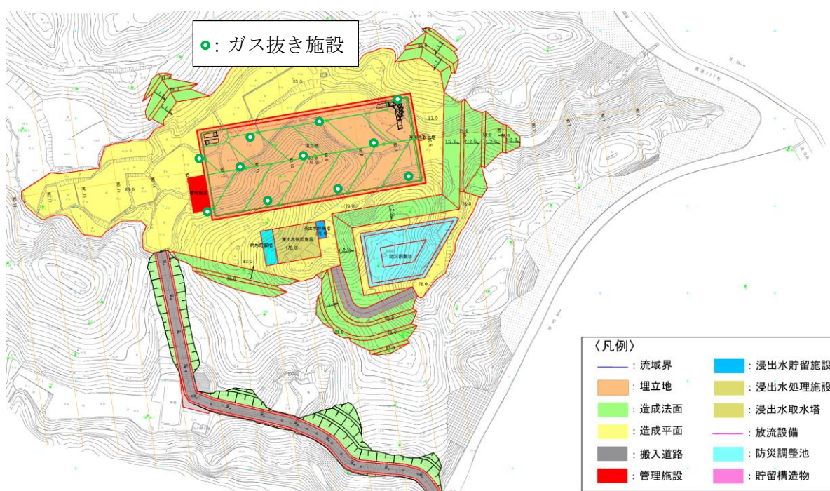
図 10.8.3 ガス抜き施設配置図
