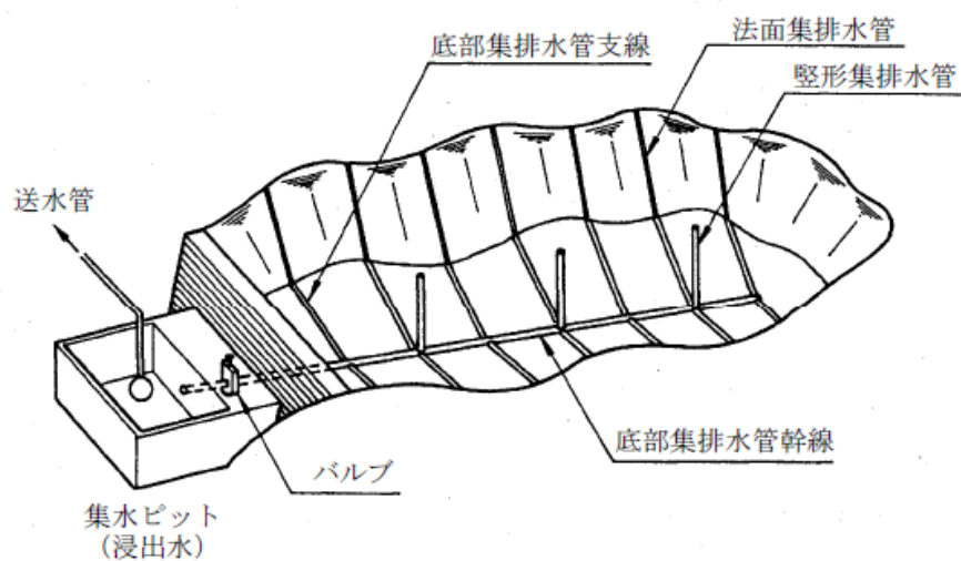
図 10.4.2 浸出水集排水施設の配置概念図
