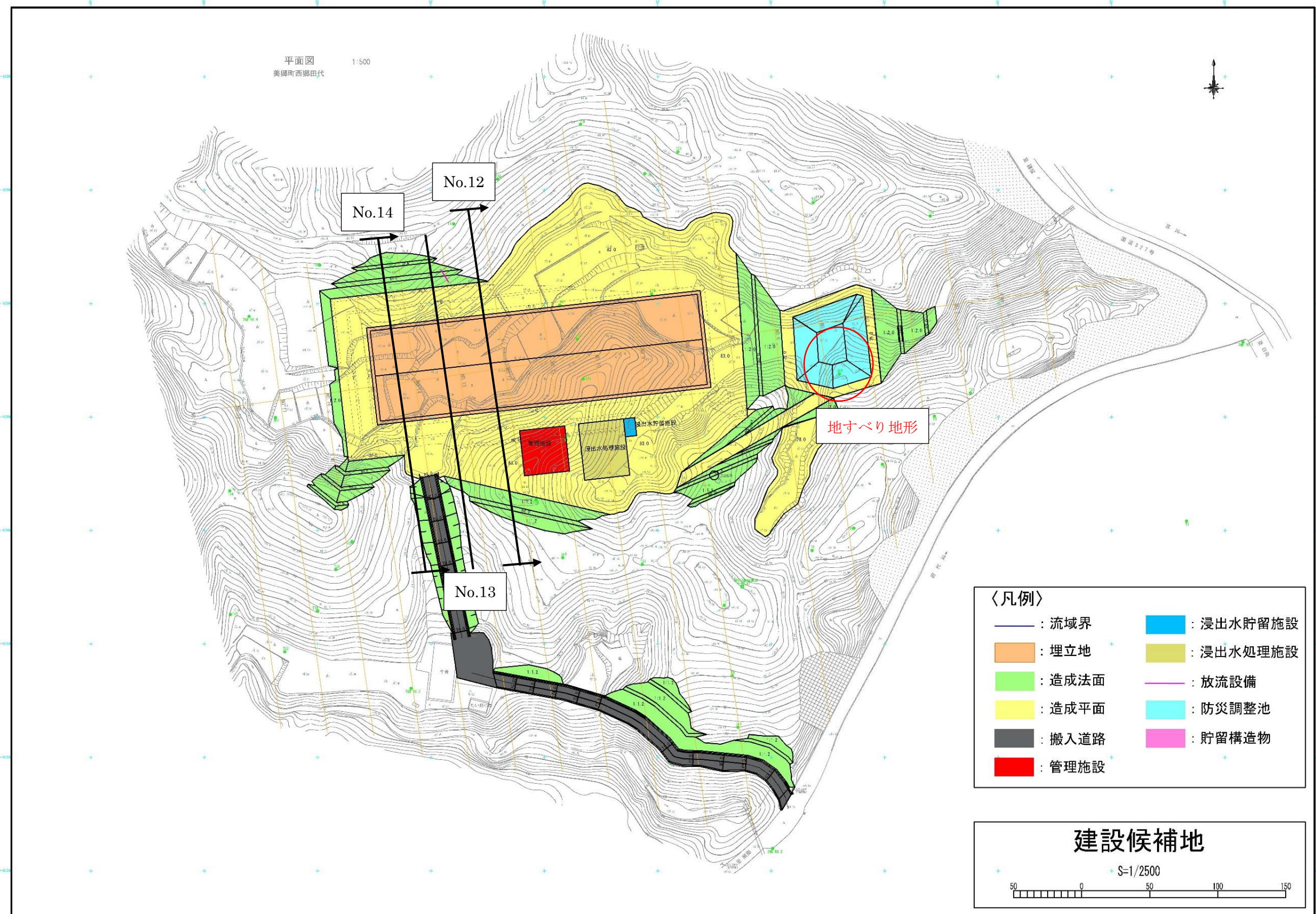
図 6.2.3 旧施設配置計画図
