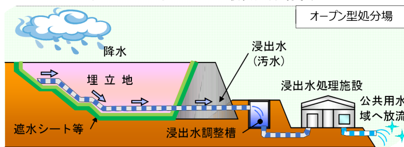
図 4.1.2 オープン型最終処分場の概要図
