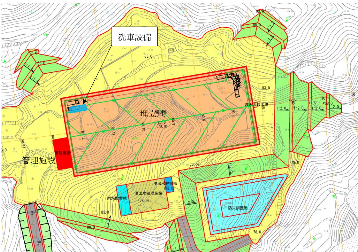
図 10.12.1 洗浄設備配置図
